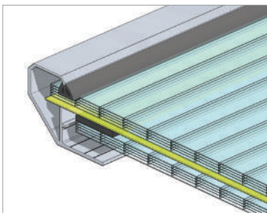
Rys. 140 Wypełnienie pasma: dwie płyty z poliwęglanu komorowego (PCA 10 + PCA 10) przedzielone pustką powietrzną (PP) i płytą NRO
