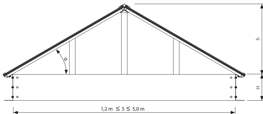
Rys. 106 Przekrój poprzeczny A-A przez świetlik piramidowy mcr PROLIGHT
