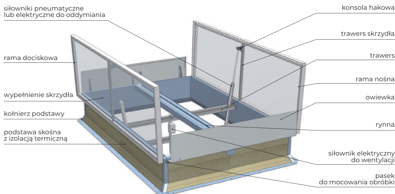
Rys. 13 Budowa kłapy oddymiającej mcr PROLIGHT DVPS wyposażonej w owiewki, z siłownikami pneumatycznymi do oddymiania oraz z siłownikiem elektrycznym do wentylacji
