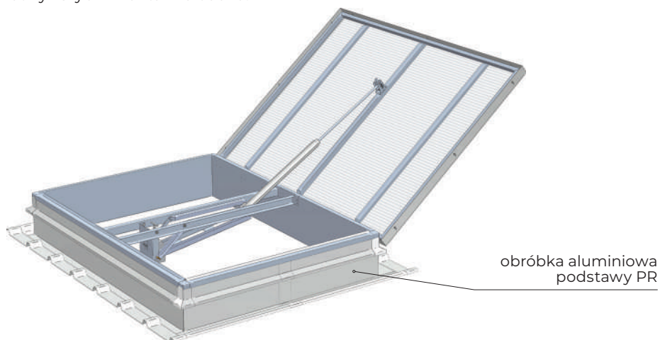
Rys. 74 Kłapa oddymiająca mcr PROLIGHT typ E z podstawą PR
