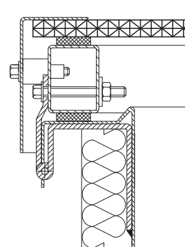
Rys. 38 Przekrój przez kłapę, wypełnienie: płyta z poliwęglanu komorowego o strukturze kratownicy
