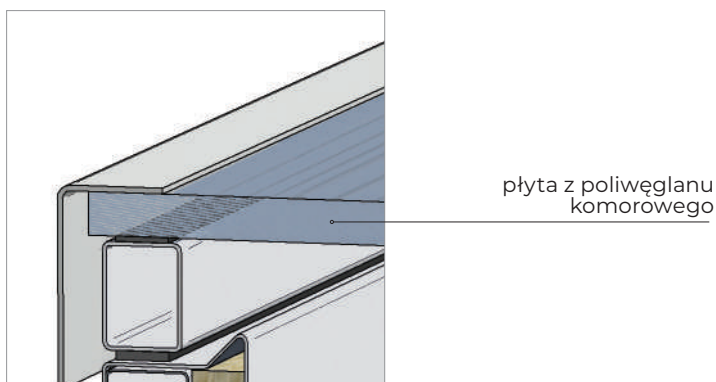
Rys. 36 Wypełnienie kłapy: płyta z poliwęglanu komorowego
