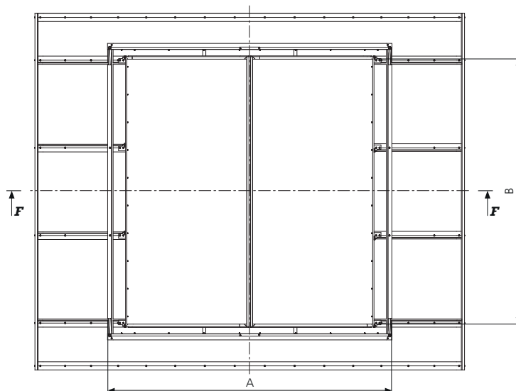
Rys. 97 Widok z góry pasma świetlnego łukowego z klapą oddymiająco-wentylacyjną jednoskrzydłową i dwuskrzydłową mcr PROLIGHT TB
