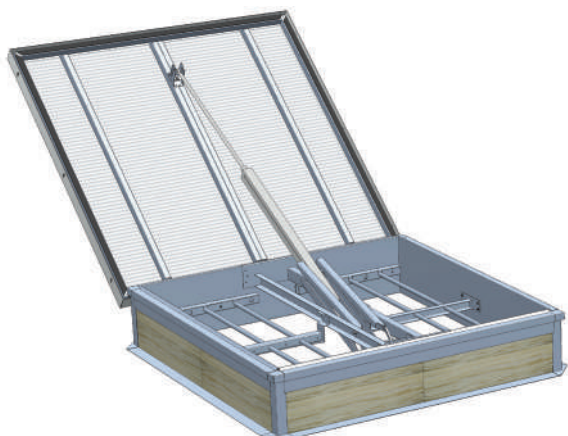
Rys. 70 Krata utrudniająca włamanie zamontowana w klapie mcr PROLIGHT typ E
