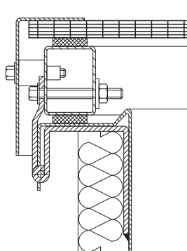
Rys. 37 Przekrój przez kłapę, wypełnienie: płyta z poliwęglanu komorowego
