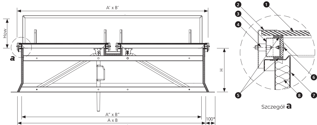
Rys. 14 Przekrój B-B przez kłapę oddymiającą mcr PROLIGHT DVPS w pozycji zamkniętej, wymiary w mm
