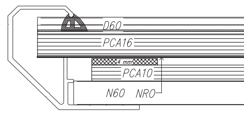
Rys. 144 Przekrój przez pasmo o szerokości 1,5÷6,0 m; rama nośna (N) i rama dociskowa (D) o szerokości 60 mm
